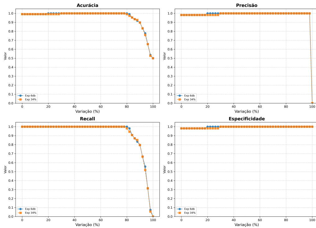
Figura 4.1: Análise de Sensibilidade entre os modelos treinados com supressão moderada (50%).
