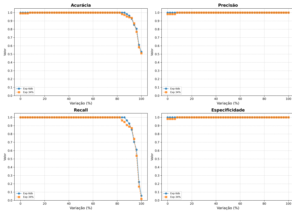
Figura 4.3: Análise dos parâmetros entre os modelos treinados com supressão moderada (50%).
