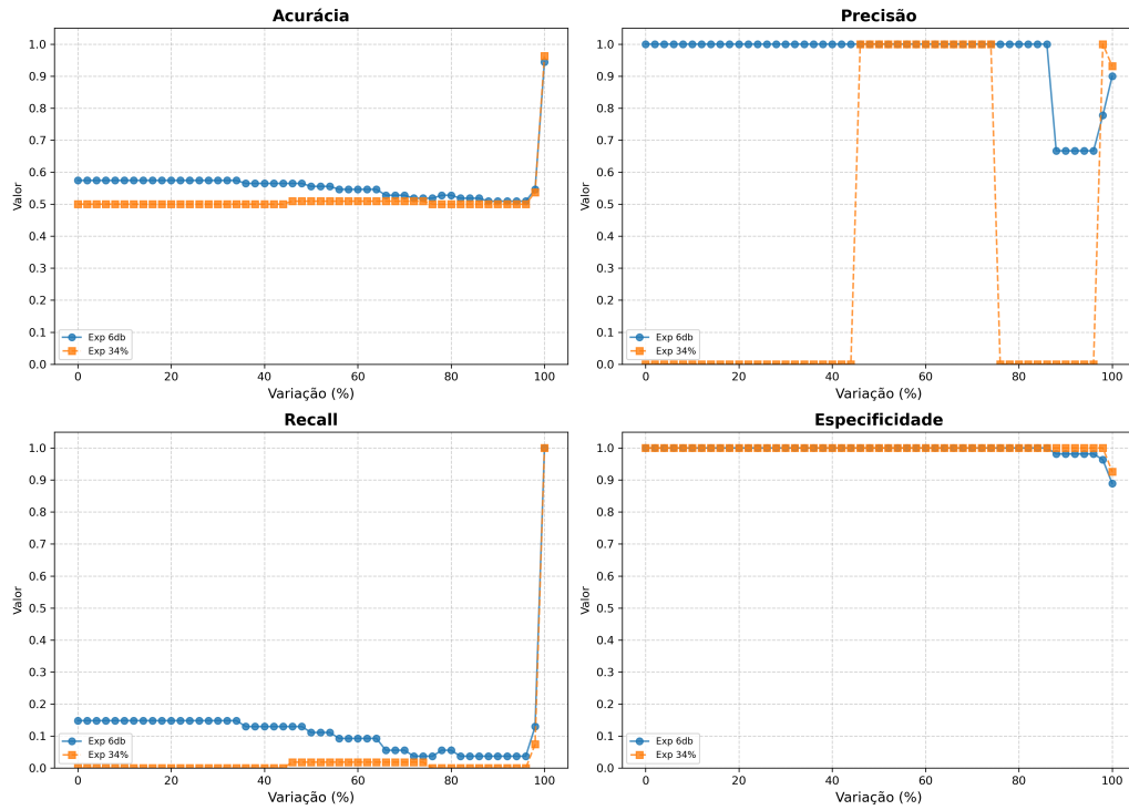
Figura 4.2: Análise de Sensibilidade entre os modelos treinados com supressão agressiva (100%).
